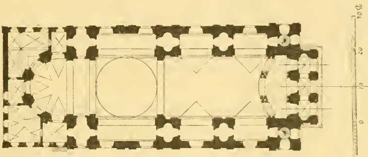
Fig. 52. Jesuitenkirche zu Mannheim. Grundriss.
